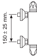
ECOTERMO DUCHA ECOTERMO SHOWER
