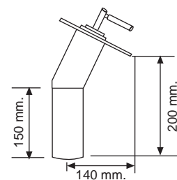
PROLONGADOR MODELOS: EXTENSION MODELS: SATELIT (ver muestra pág. 20) INOX PLATONIC PLATINUM
